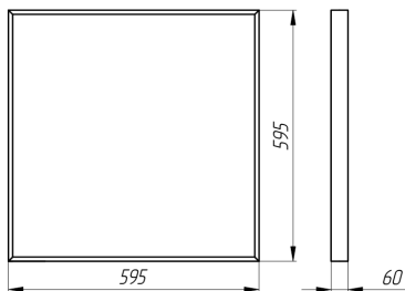
Рисунок 2 — Габаритные размеры светильников Office Comfort 595x595x60.
